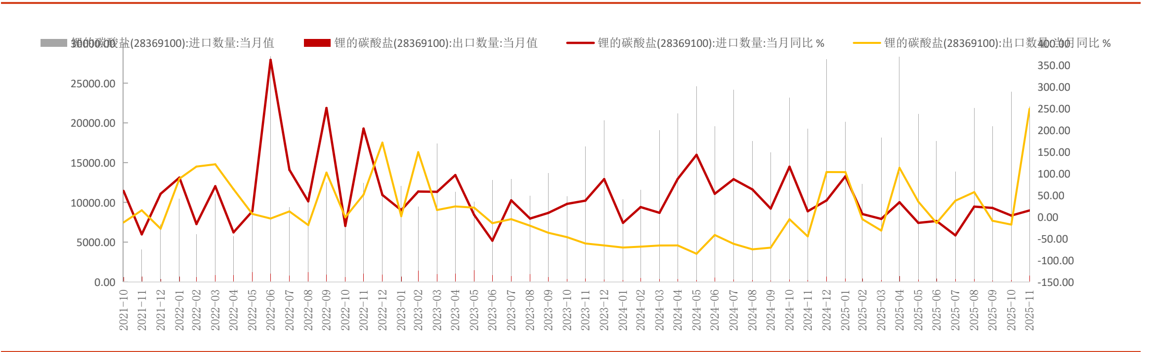
图4：碳酸锂进出口及增速
